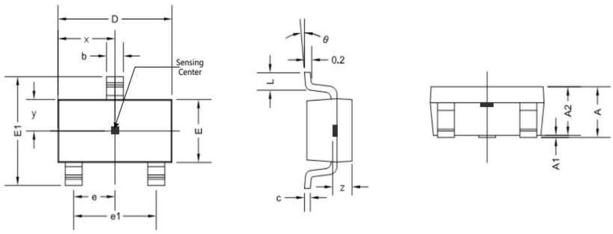
SOT23-3L 封装尺寸
