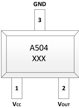
SOT23 (Thin) / SOT23-3L
