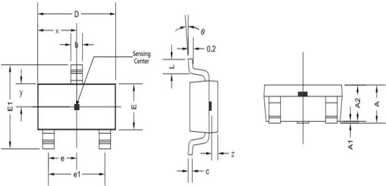
SOT23（Thin Outline）封装尺寸
